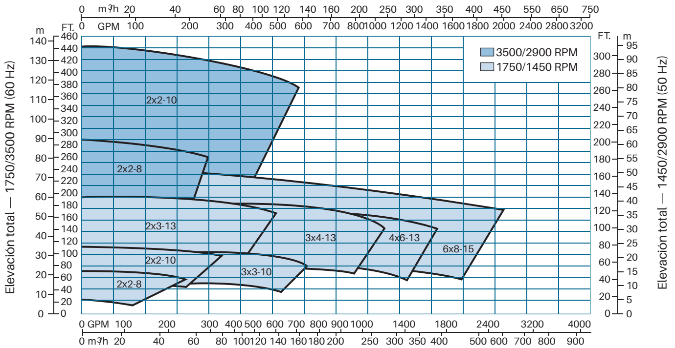
Capacidad — 1750/3500 RPM (60 Hz)
