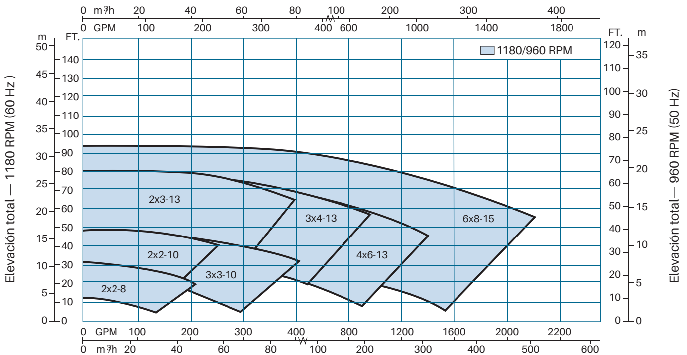
Capacidad — 1180 RPM (60 Hz)
